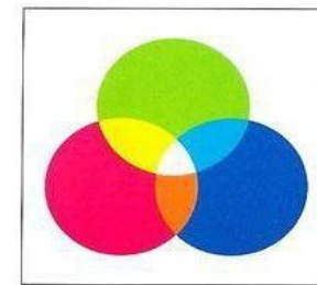
Synthèse additive
