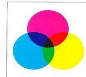
Synthèse soustractive
